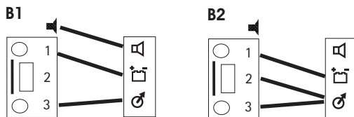
Варианты установки со стереофонической аудиосистемой
