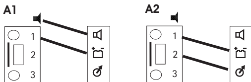
Варианты установки с монофонической аудиосистемой
