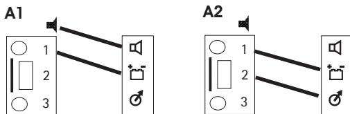
Варіанти встановлення для відтворення звуку в режимі моно
