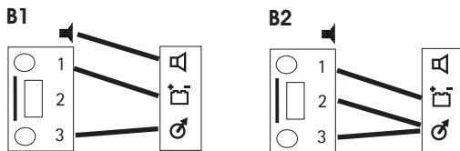
Варіанти встановлення для відтворення звуку в режимі стерео
