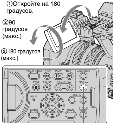
Кнопка DISPLAY
